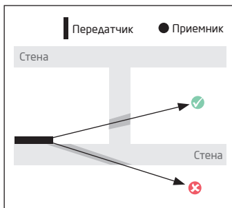
Рис. нр. 4 Проникновение радиосигнала в помещении
