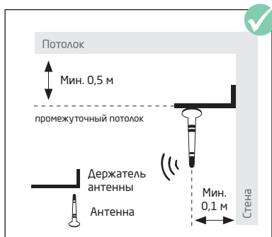
Рис. нр. 7 Правильная установка антенны под потолком
