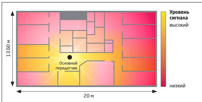
Рис. нр. 5 Распространение радиосигнала в здании
