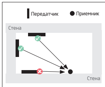
Рис. нр. 6 Особенности установки антенны
